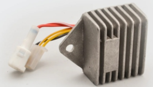
Rectifier
